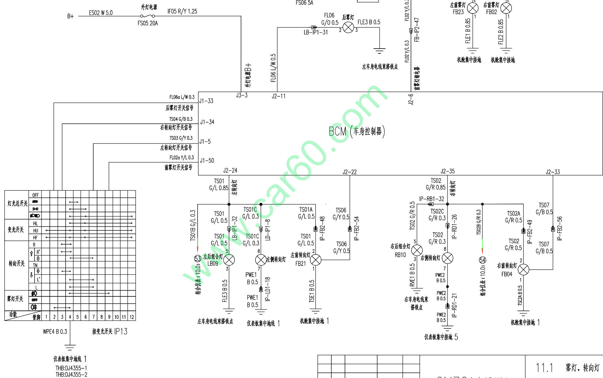
CM7C电气原理图
